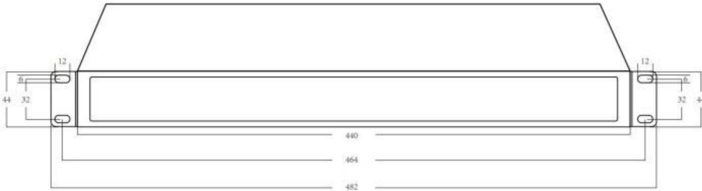
机架式挂耳
