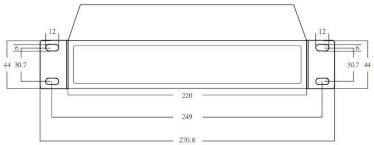
壁挂式挂耳
