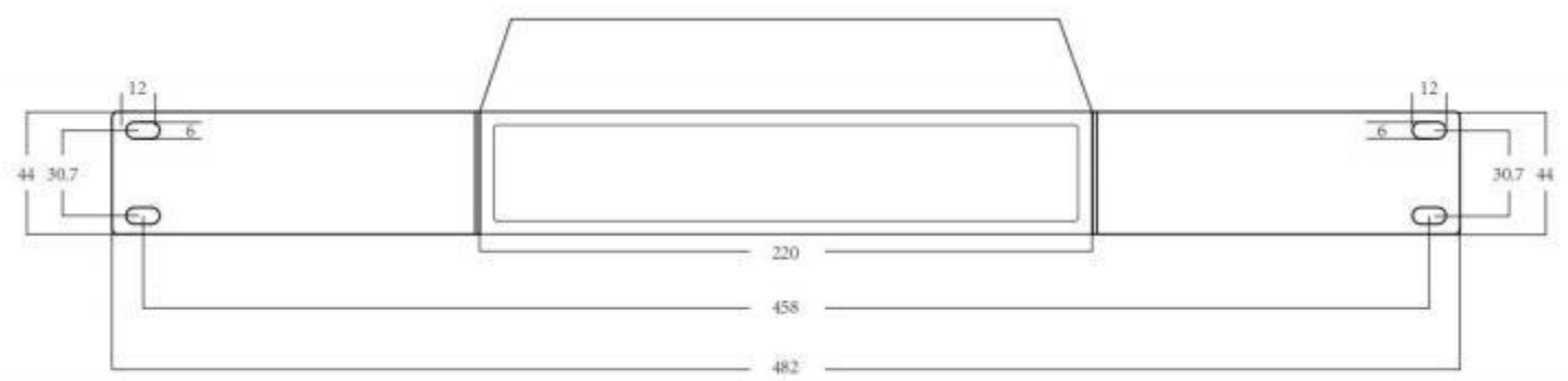
机架式挂耳
