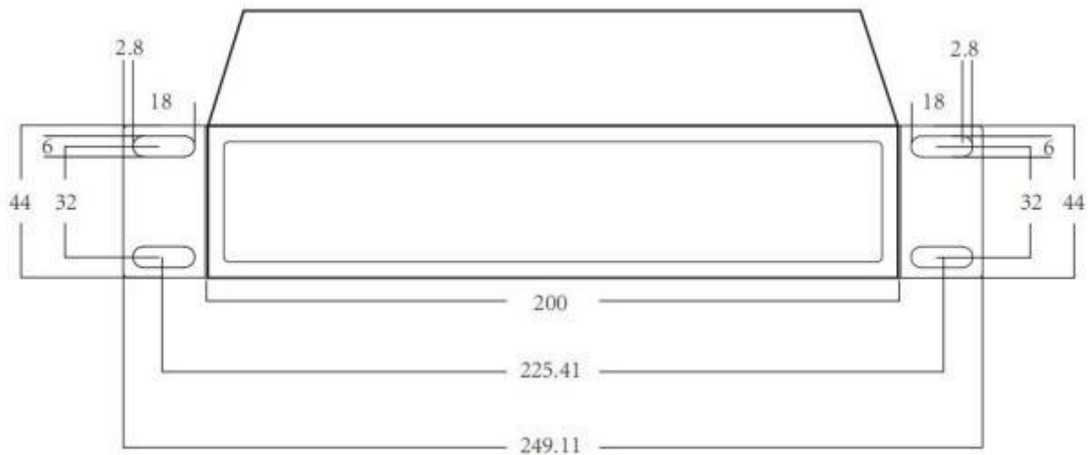
壁挂式挂耳
