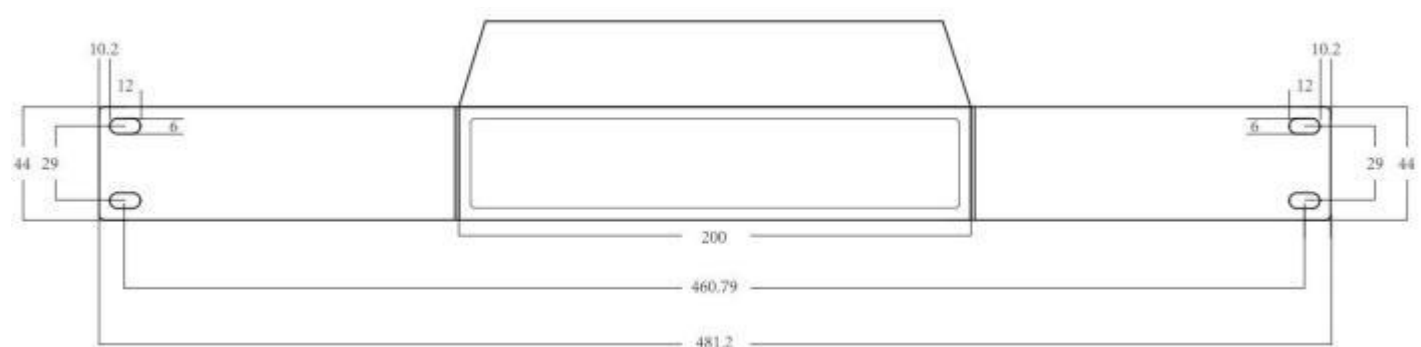
机架式挂耳
